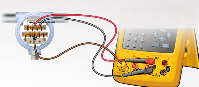
Conexión de calibración del transmisor TC
