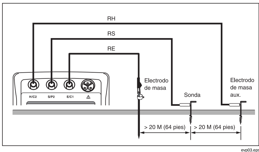
Figura 4. Configuración de la medición de tres polos
