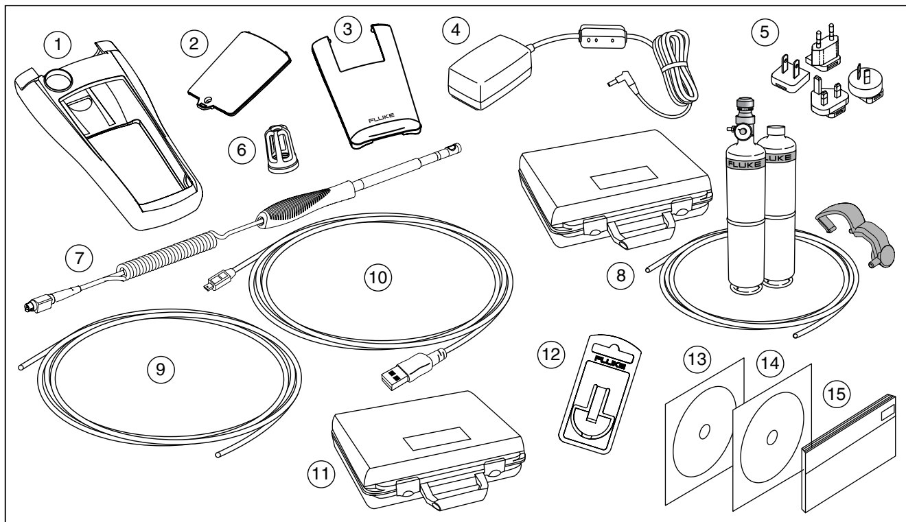
Figura 6. Accesorios y repuestos reemplazables
