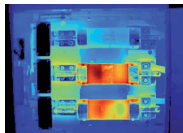
Cuadro eléctrico trifásico con desequilibrio de carga
