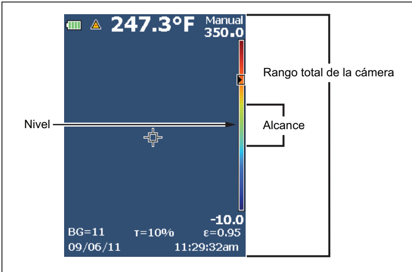
Figura 3. Configuración del nivel y el alcance
