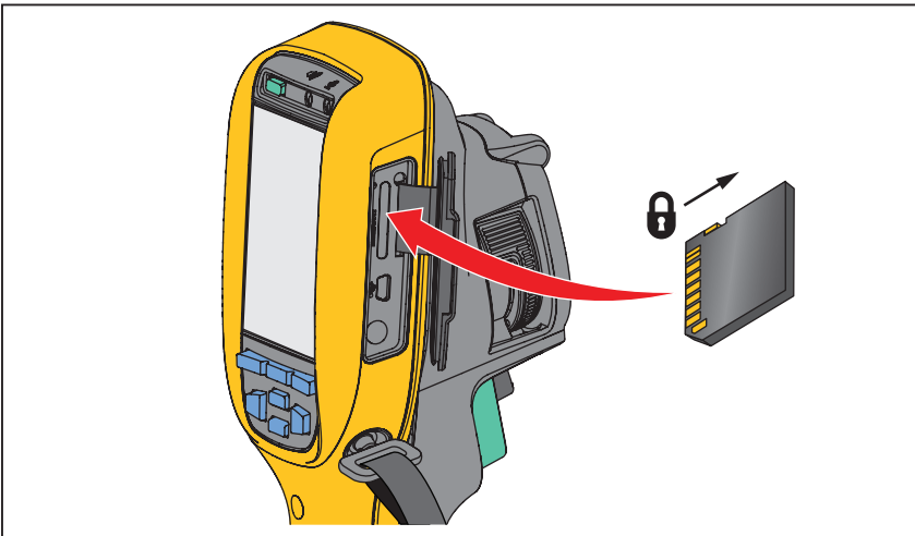
Figura 2. Inserción y extracción de la tarjeta de memoria SD
