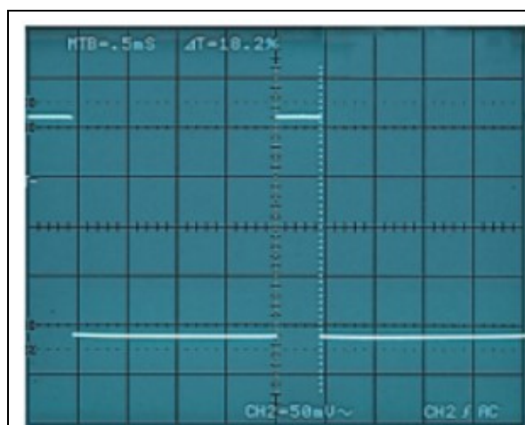
Fig. 1a Analog Oscilloscope
